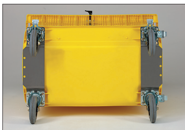
Bodemplaten, versteviging ten behoeve van UN-keur.
